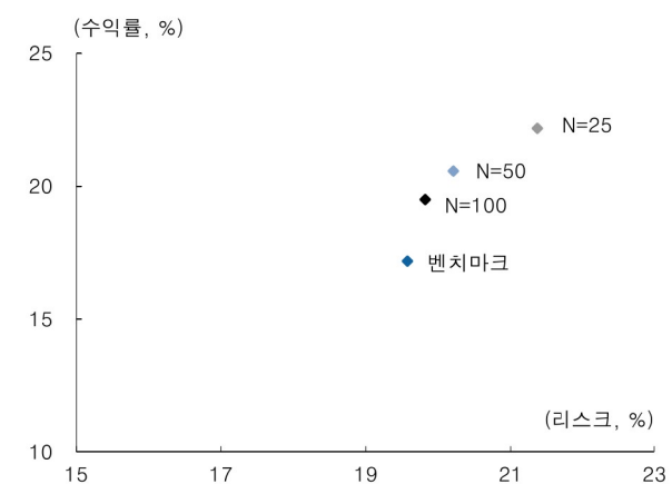
[그림 26] 종목수에 따른 수익률과 리스크
