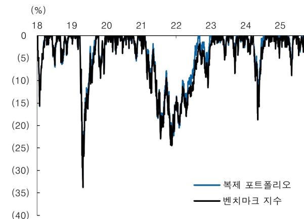
[그림 12] 벤치마크 지수와 복제 포트폴리오 Drawdown 추이
