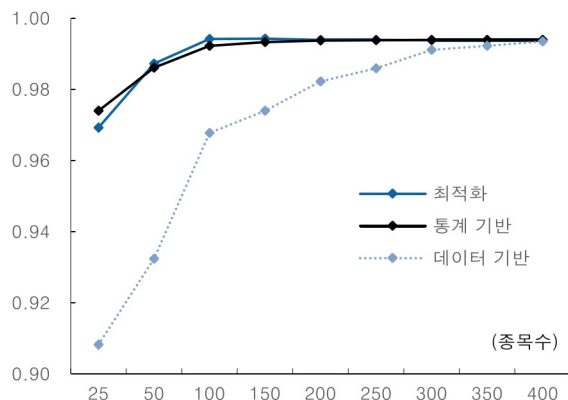
[그림 27] 종목수에 따른 상관계수 변화
