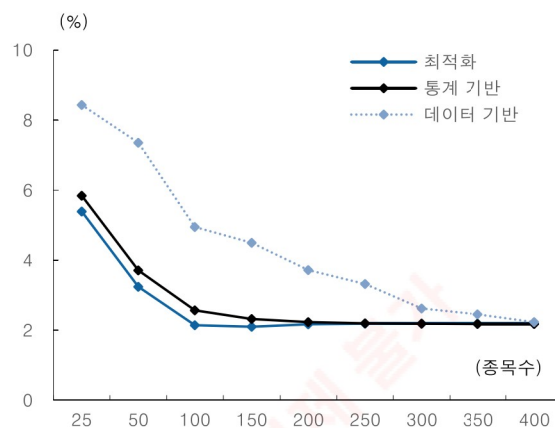
[그림 28] 종목수에 따른 연환산 추적오차 변화
