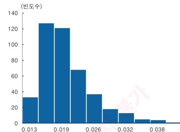
[그림 4] S&P500 지수 구성종목의 일간 표준편차 분포
