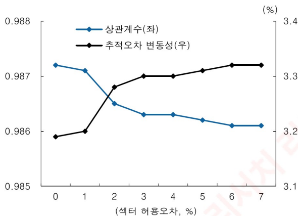
[그림 29] 섹터 중립 조건하의 상관도와 추적오차 변동성
