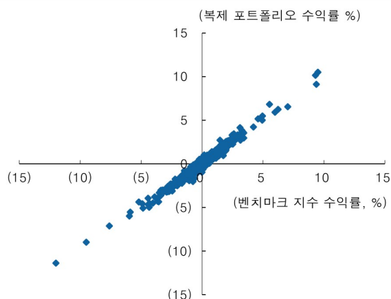
[그림 9] 벤치마크 지수와 복제 포트폴리오 수익률 산포도
